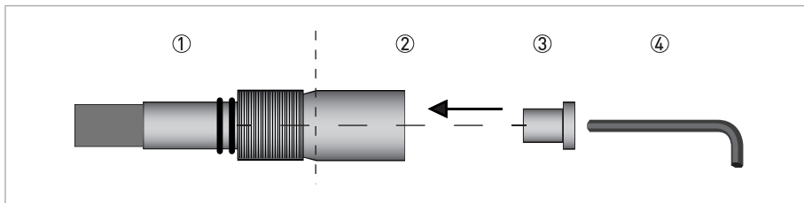
Рисунок 8-24: Установите бронзовую фиксирующую гайку.
