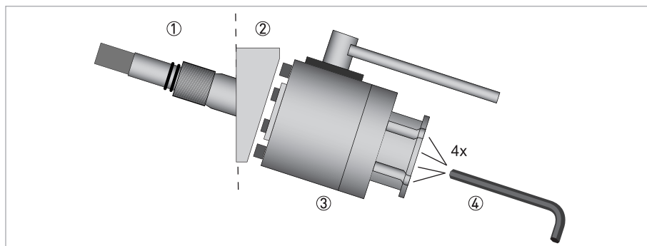
Рисунок 8-27: Установите шаровой кран извлекающего устройства на расходомер.
