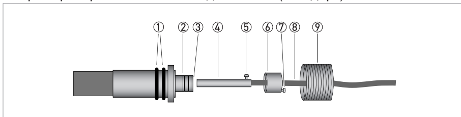
Рисунок 8-3: Сенсор в сборе
