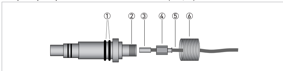
Рисунок 8-4: Сенсор в сборе
