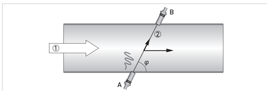
Рисунок 9-1: Принцип измерения времени прохождения
