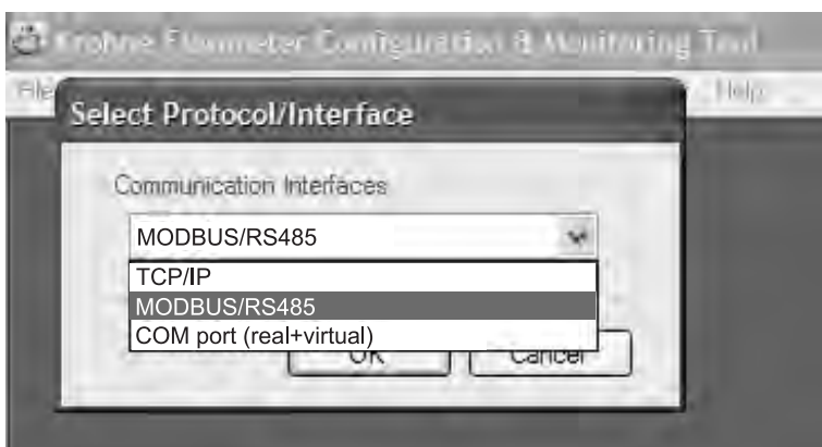
Рисунок 7-4: Интерфейсы связи
