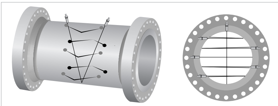
Рисунок 9-4: Схема с несколькими акустическими каналами
