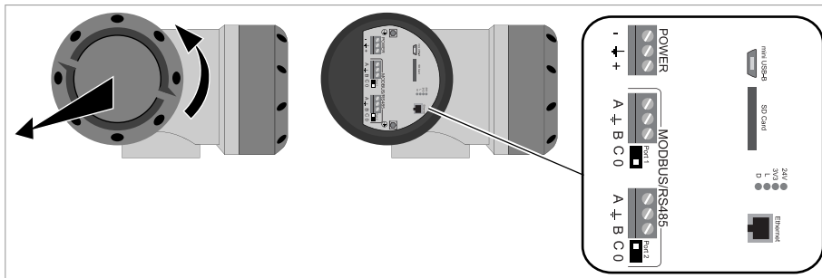
Рисунок 4-2: Подключение последовательной передачи данных
