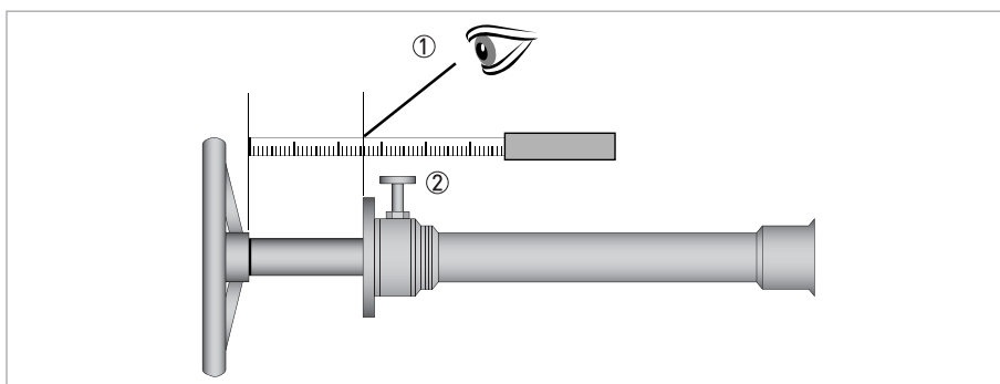
Рисунок 8-32: Измерьте длину вала.
