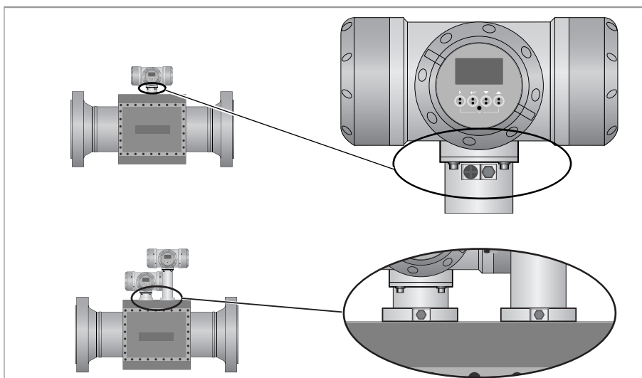
Рисунок 4-6: Местоположение контакта заземления
