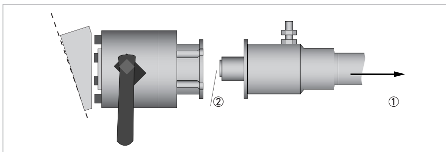
Рисунок 8-36: Снимите трубу.
