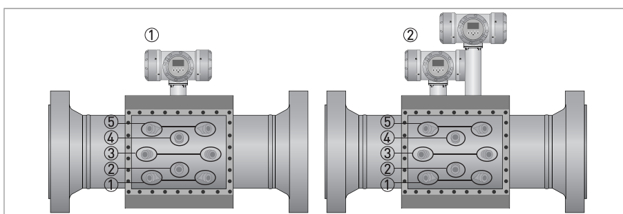
Рисунок 2-2: Местоположение датчиков и блока электроники
