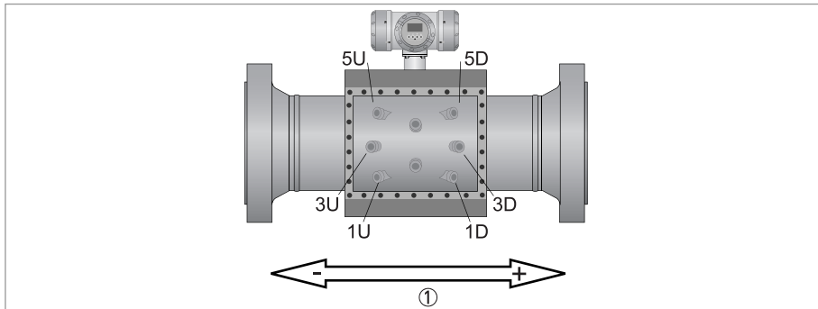
Рисунок 8-18: Преобразователи сигнала на передней стороне расходомера
