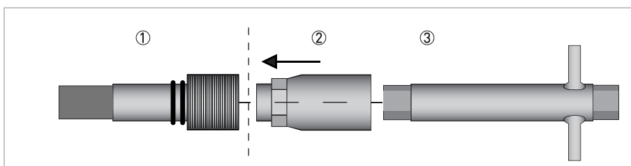
Рисунок 8-23: Установите переходник измерительного преобразователя.
