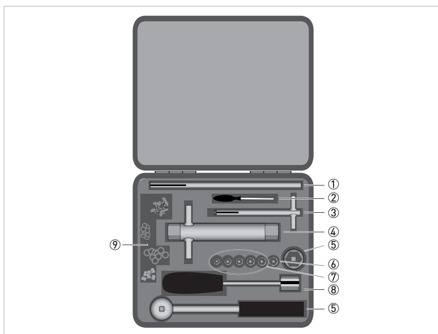
Рисунок 8-1: Программный инструментарий
