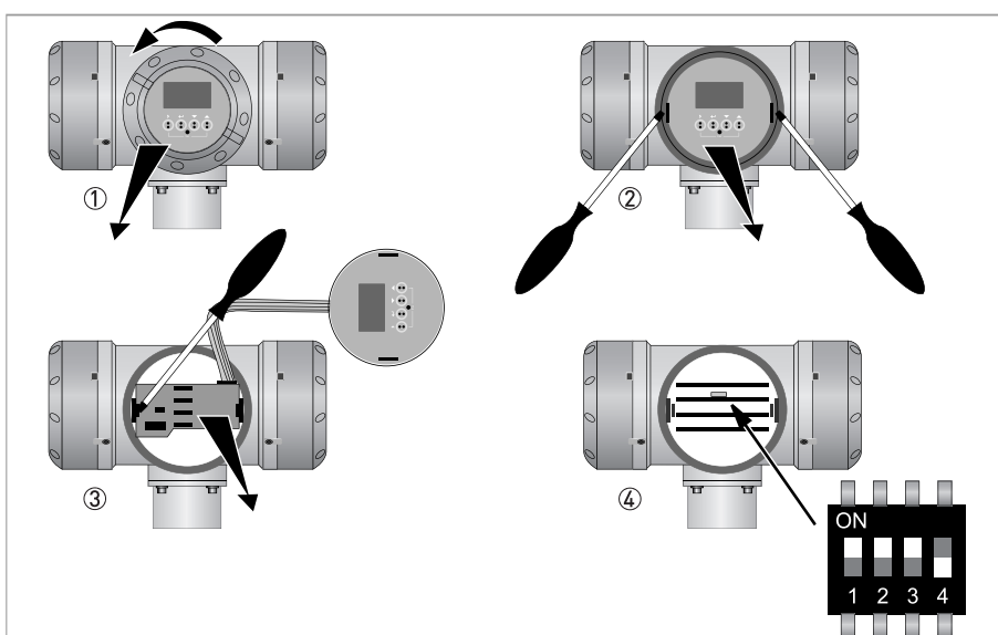
Рисунок 6-3: Местоположение переключателя DIP для пломбирования
