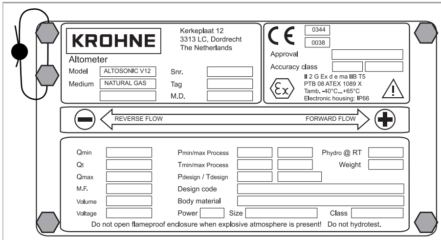
Рисунок 6-4: Уплотнение типовой таблички
