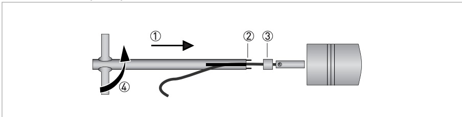
Рисунок 8-7: Снимите крышку.
