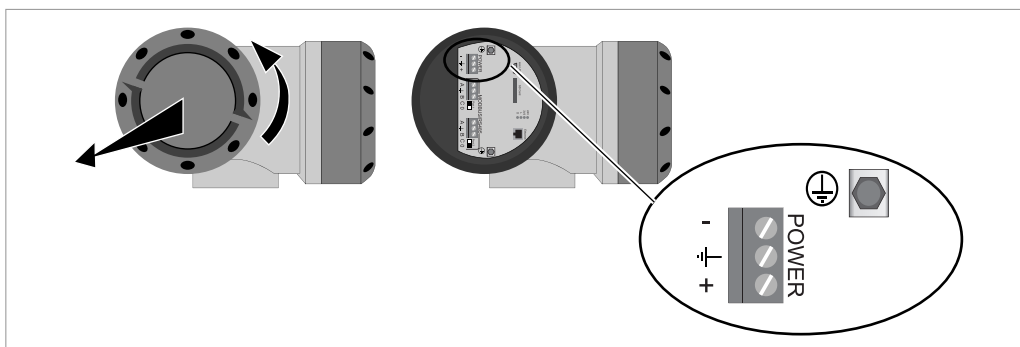
Рисунок 4-4: Местоположение цепей для подключения питания
