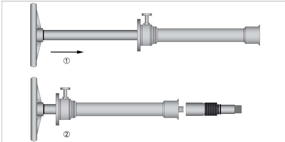
Рисунок 8-37: Извлеченный измерительный преобразователь
