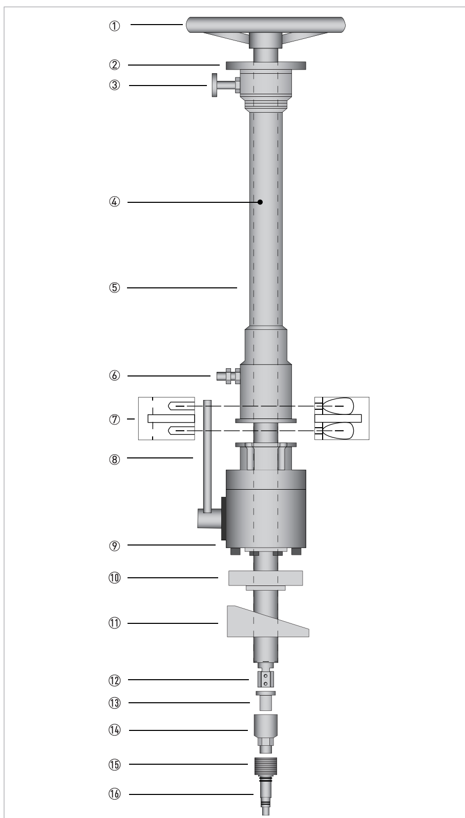
Рисунок 8-17: Съемник
