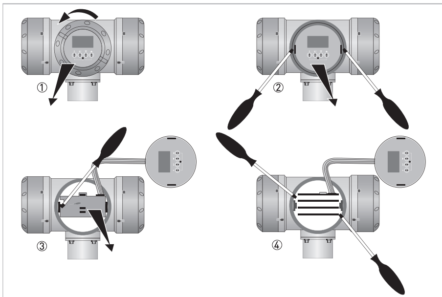
Рисунок 8-38: Приготовьтесь снять блок электроники
