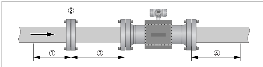
Рисунок 3-4: Необходимы прямые участки на входе и выходе
