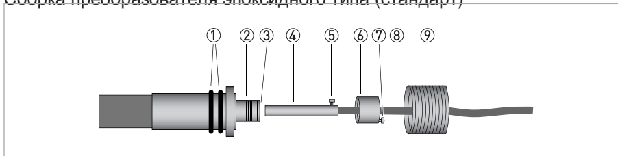
Рисунок 2-3: Сенсор в сборе
