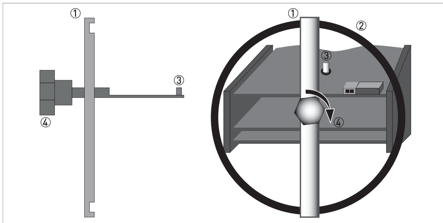
Рисунок 8-39: Используйте выталкиватель, чтобы освободить электронный блок из разъема
