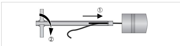
Рисунок 8-15: Установка Ex-d-сертифицированных разъема и колпачка
