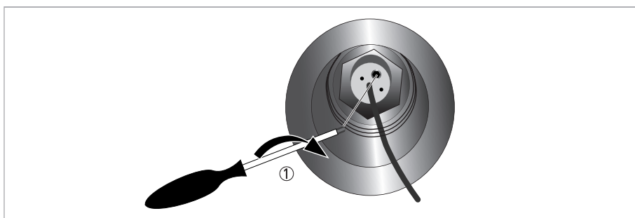
Рисунок 8-16: Затяните фиксирующий винт M2
