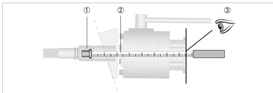
Рисунок 8-28: Измерьте глубину.
