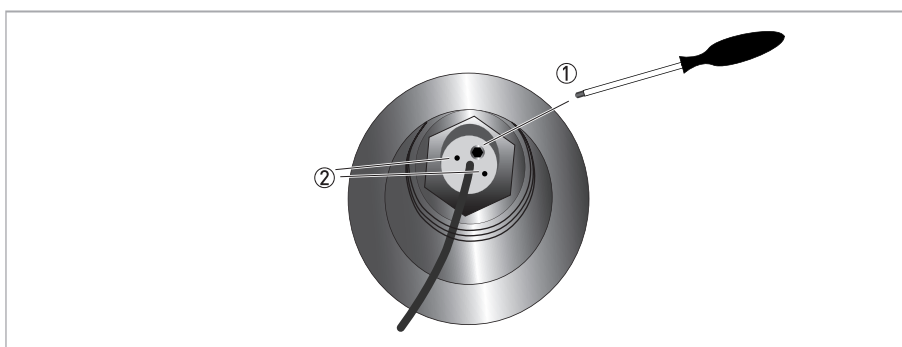
Рисунок 8-6: Вид на установленный измерительный преобразователь
