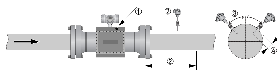
Рисунок 3-5: Местоположение датчиков температуры и давления
