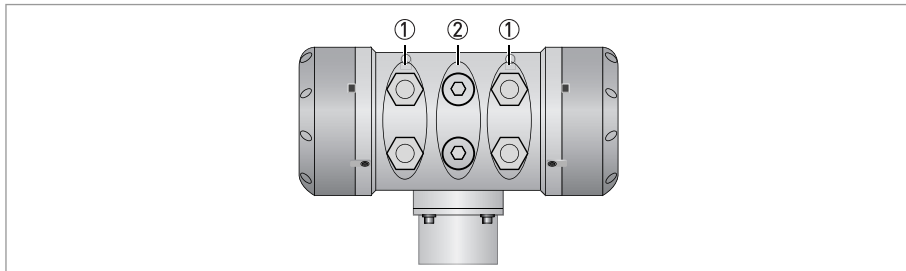
Рисунок 4-5: Расположение кабельных вводов
