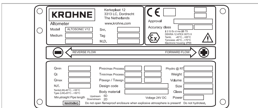
Рисунок 2-6: Пример типовой таблички ATEX
