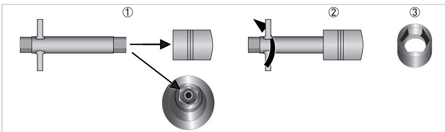
Рисунок 8-9: Снятие гайки измерительного преобразователя
