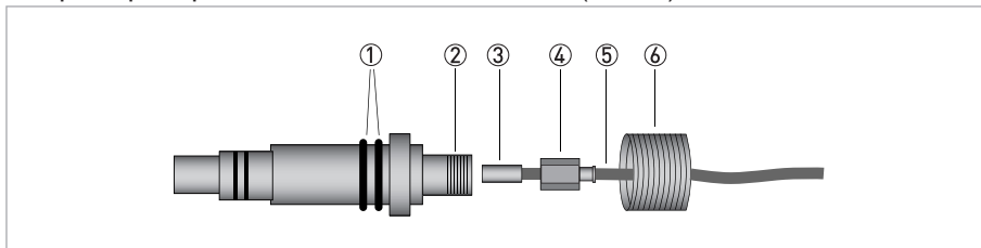
Рисунок 2-4: Сенсор в сборе
