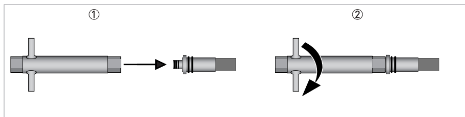
Рисунок 8-12: Установка измерительного преобразователя в инструмент
